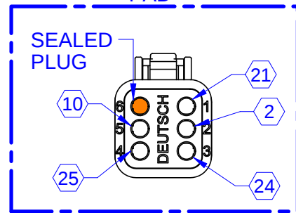
VIEW B DEUTSCH DT06-6S CONTACT 1062-16-0122 WEDGELOCK W6S SEAL PLUG 0413-217-1605
