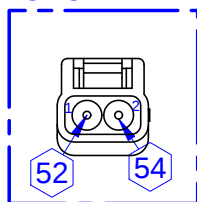
VIEW I DEUTSCH DTM06-2S CONTACT 1062-20-0122 WEDGELOCK WM-6S
